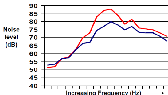
Figura nr 3: Reducerea la sursă Diminuarea nivelului de zgomot în funcție de frecvență, suprapusă peste caracteristica de frecvență a unui tren.
