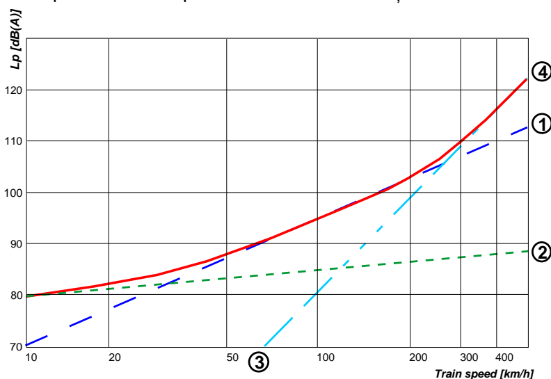
Figura nr 2: Dependenta nivelului de zgomot al unui tren, ca rezultat al compunerii nivelurilor de zgomot ale diferitelor surse în funcție de viteză: 1- Zgomotul de rulare; 2 - Zgomotul de tracțiune; 3 - Zgomotul aerodinamic; 4 - Zgomotul total
