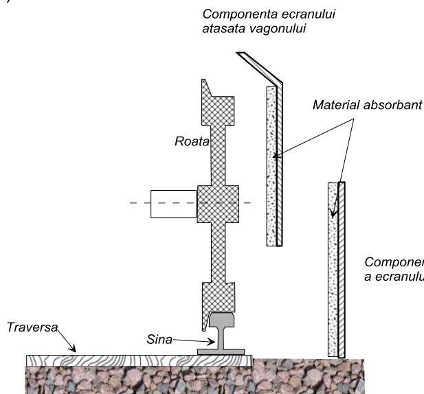
Figura nr 6: Schița unui ecran combinat – partea superioară este atașată vagonului, iar partea inferioară, de înălțime mică este situată în vecinătatea căii de rolare, în zona unde este necesară protecția.
